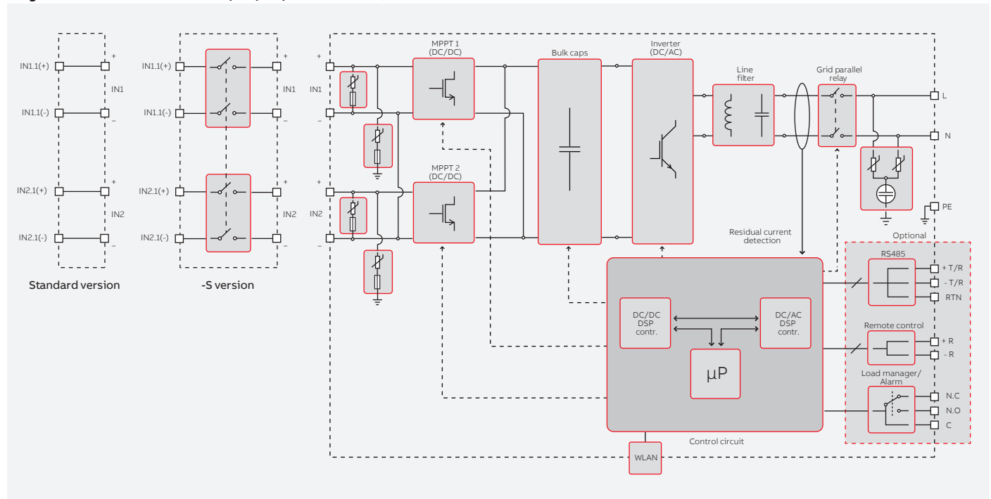
Diagramma a blocchi UNO-DM-3.3/4.0/4.6/5.0-TL-PLUS-Q
